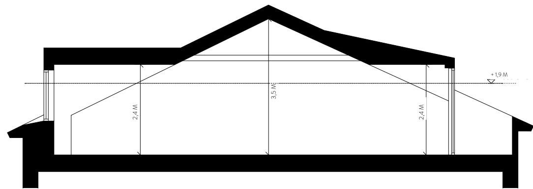
TVÄRSNITT
