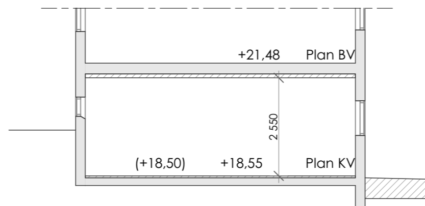
SEKTION B-B SKALA 1:100
