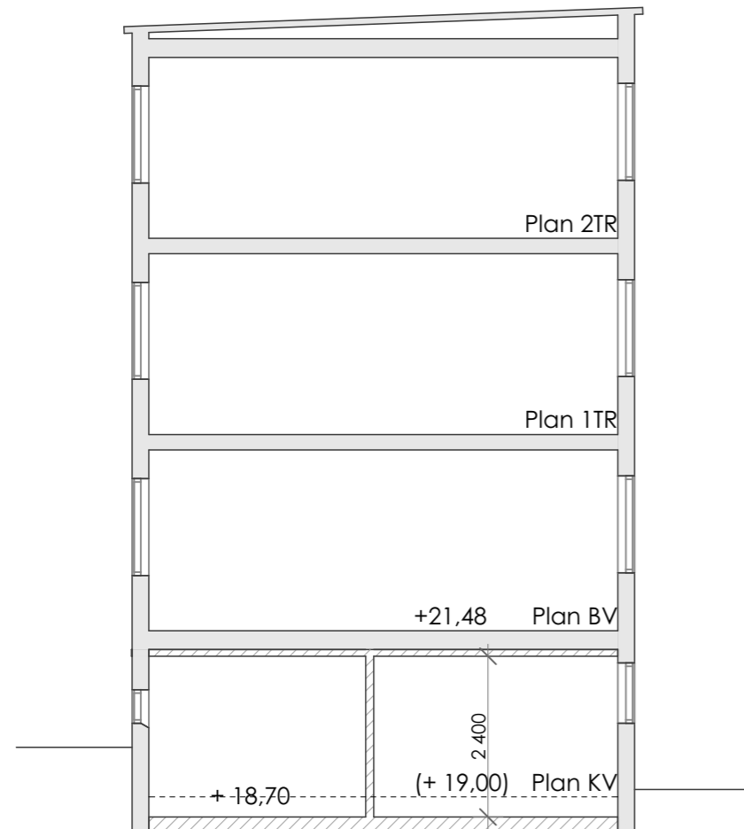
SEKTION A-A SKALA 1:100
