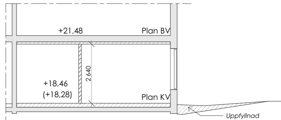
SEKTION C-C SKALA 1:100
