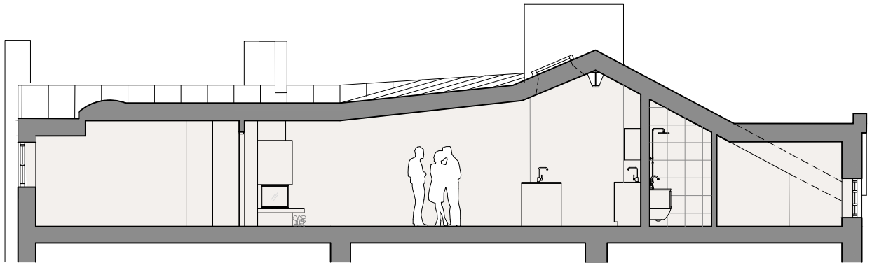
SEKTION B - B
