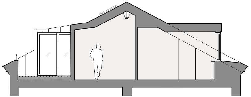
SEKTION A - A
