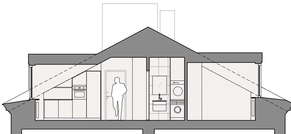
SEKTION B - B
