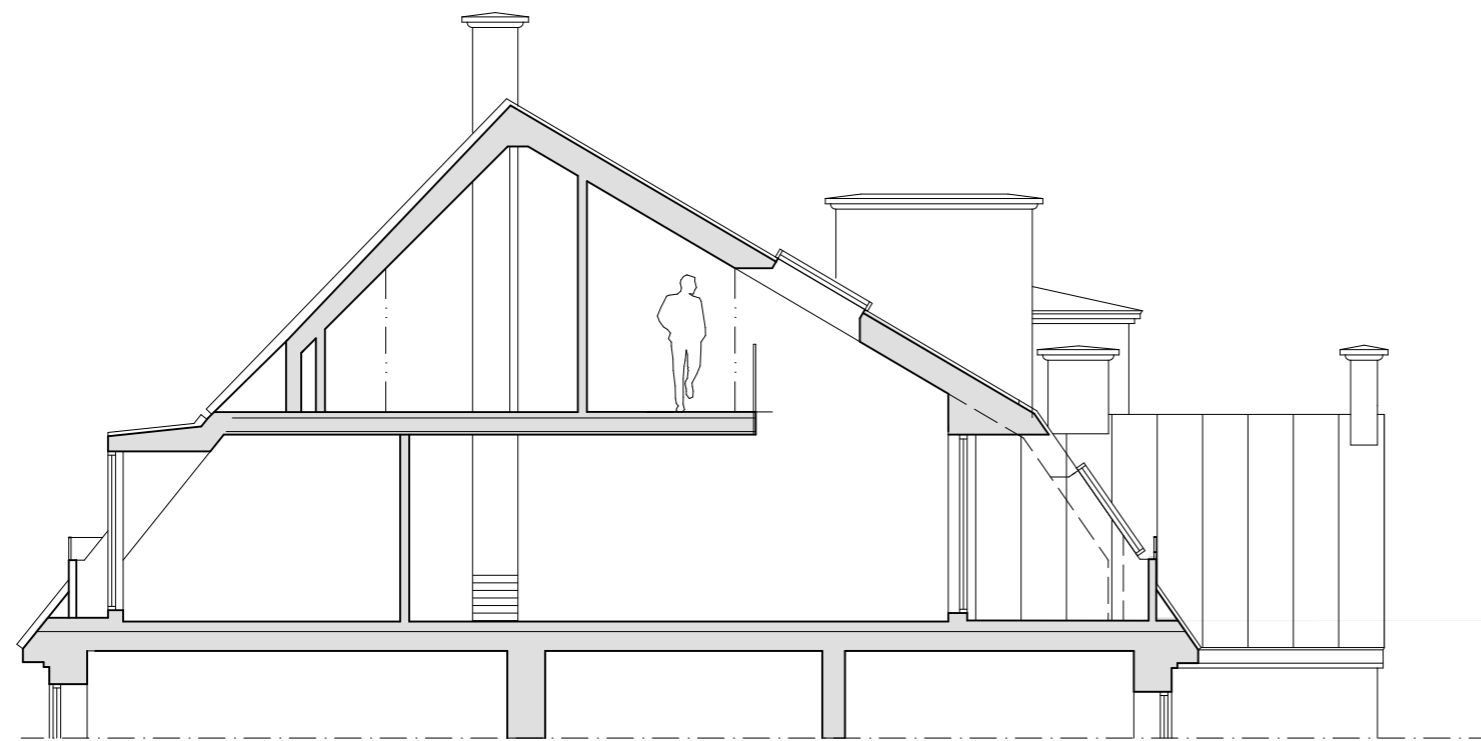
SEKTION B-B SKALA 1:100
