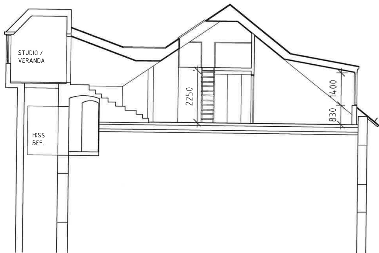
C-C
