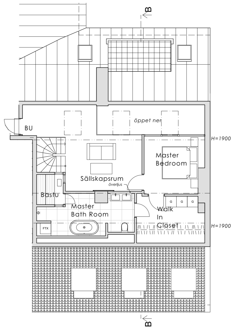
LOFT SKALA 1:100
