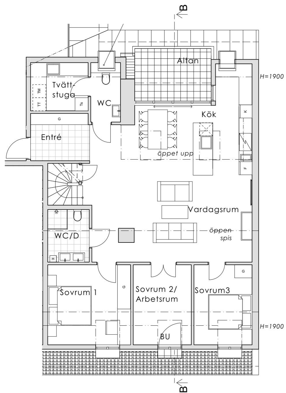
VINDSPLAN SKALA 1:100
