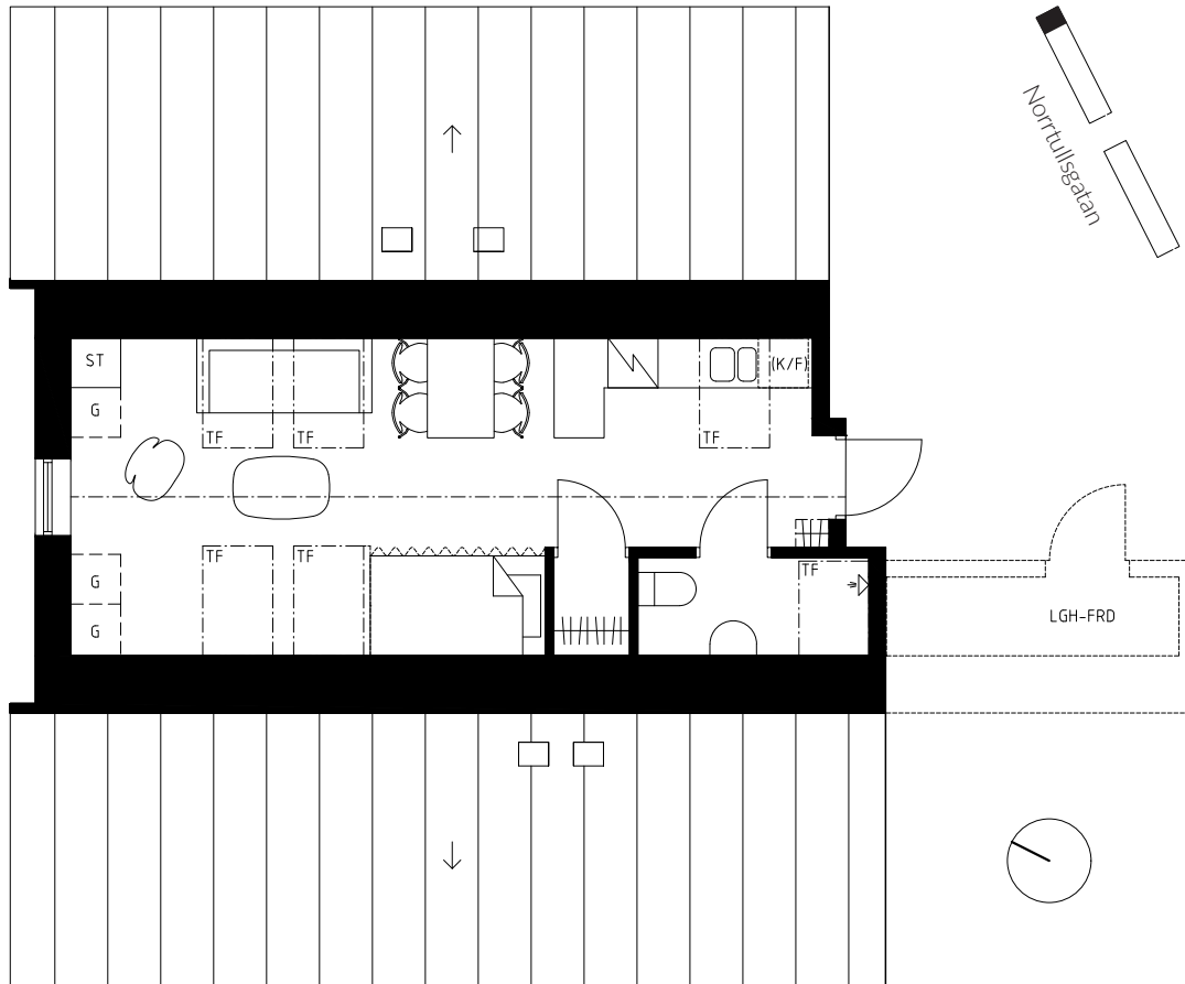
Planritning 1:100
