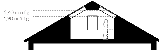
Principsektion 1:200 (A4)
